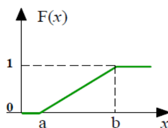
Fonction de répartition
