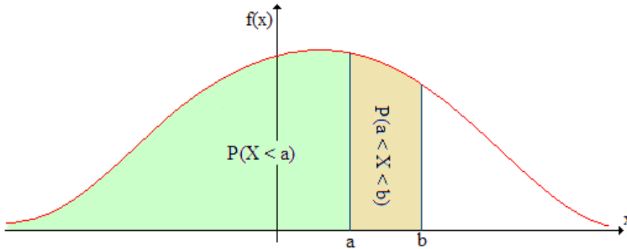
FIGURE 7.1 : Densité de probabilité
