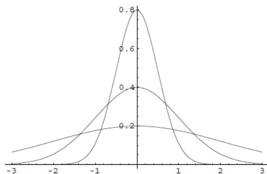
Espérances identiques, écarts types 0.5, 1, 2 différents
