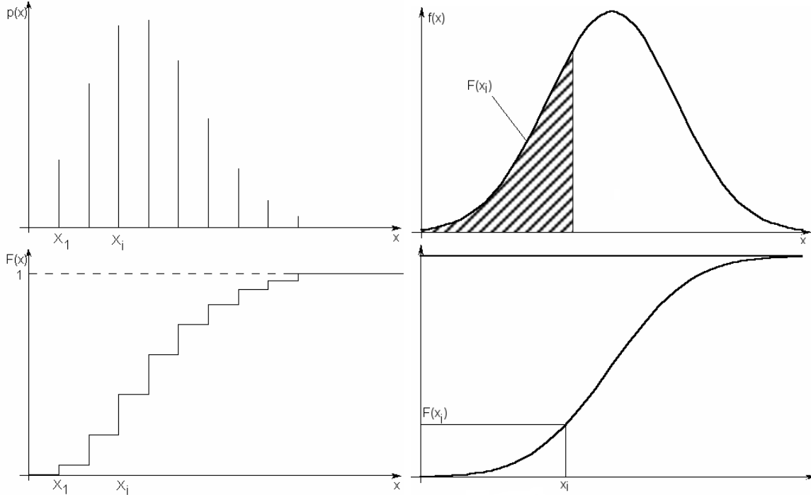
FIGURE 7.2 : Lois de probabilité et fonction de répartition (variables discrètes et continues)
