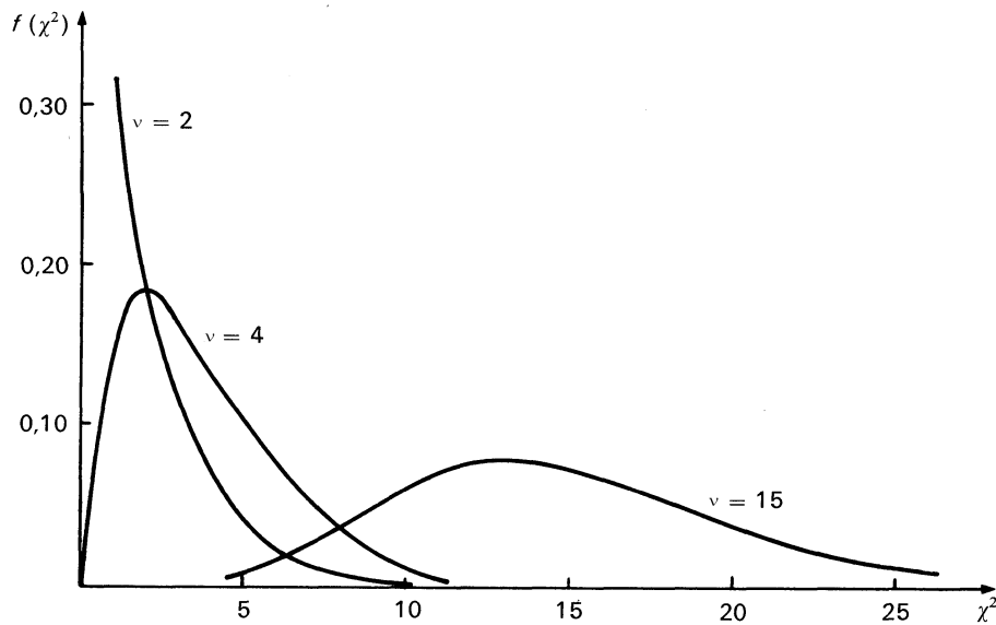
Forme de la loi du \chi^2 suivant le nombre \nu de degrés de liberté
