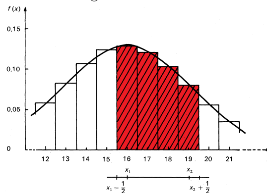
Histogramme binomial et courbe normale.
