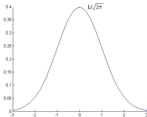
Forme de la loi normale : courbe de densité de la variable normale centrée réduite
