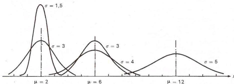
Courbes de densité de probabilité de la variable normale
