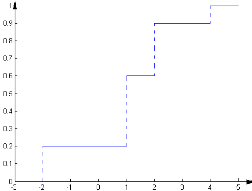
FIGURE 5.1 : Fonction de répartition
