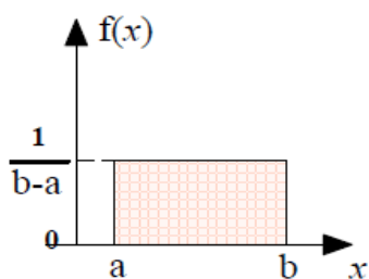
Fonction de densité de probabilité
