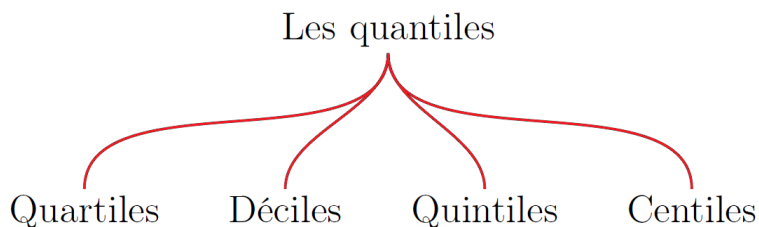
FIGURE 7.3 : Diagramme des différents quantiles
