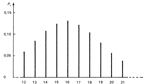
Diagramme en bâtons
