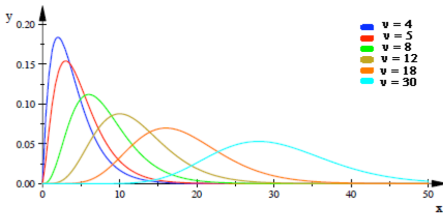
Densité de \chi^2 pour \nu = 4, 5, 8, 12, 18, 30 .
