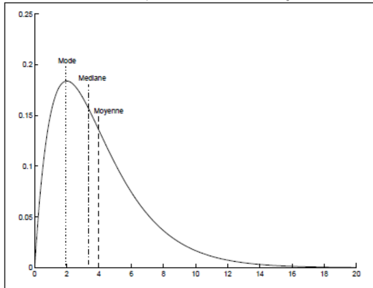
FIGURE 7.4 : Le mode, la médiane et la moyenne d'une loi
