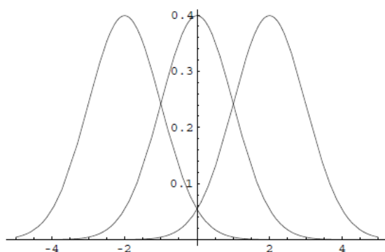
Ecart types identiques, espérances -2, 0, 2 différentes
